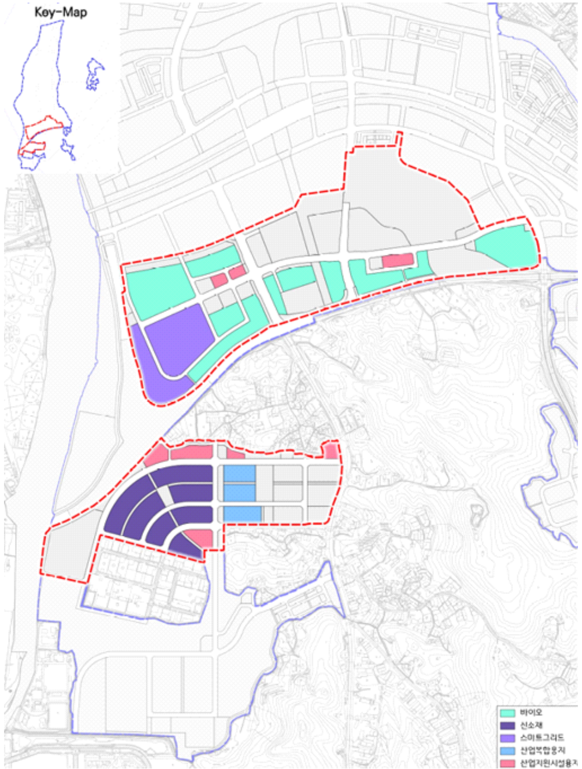
그림 3-2 왕숙도시첨단산업단지 배치계획
